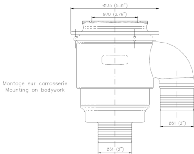
Accoupleur Femelle
